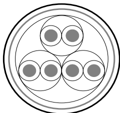
3对电缆的结构图例
